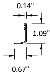
⑨ GLAZING IG
