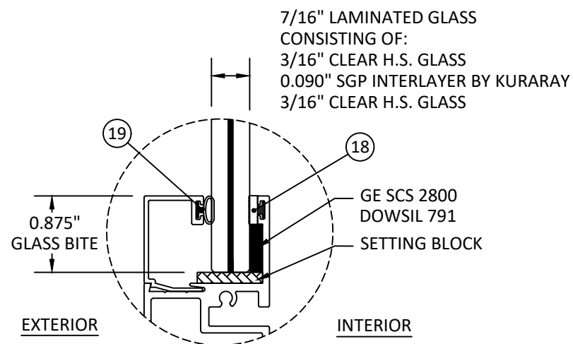
GLAZING DETAIL G2
