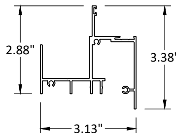
② JAMB
