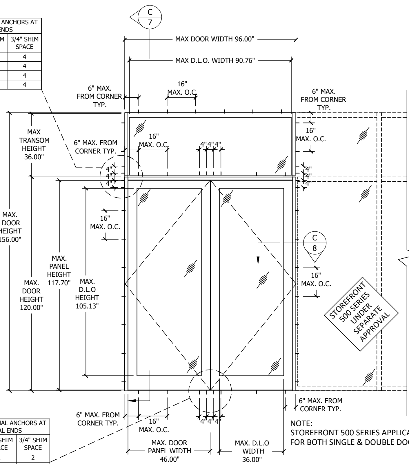
ELEVATION
