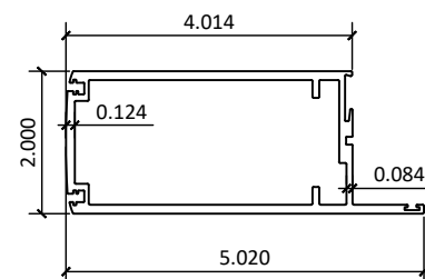
9 600-10 - DOOR STILE
