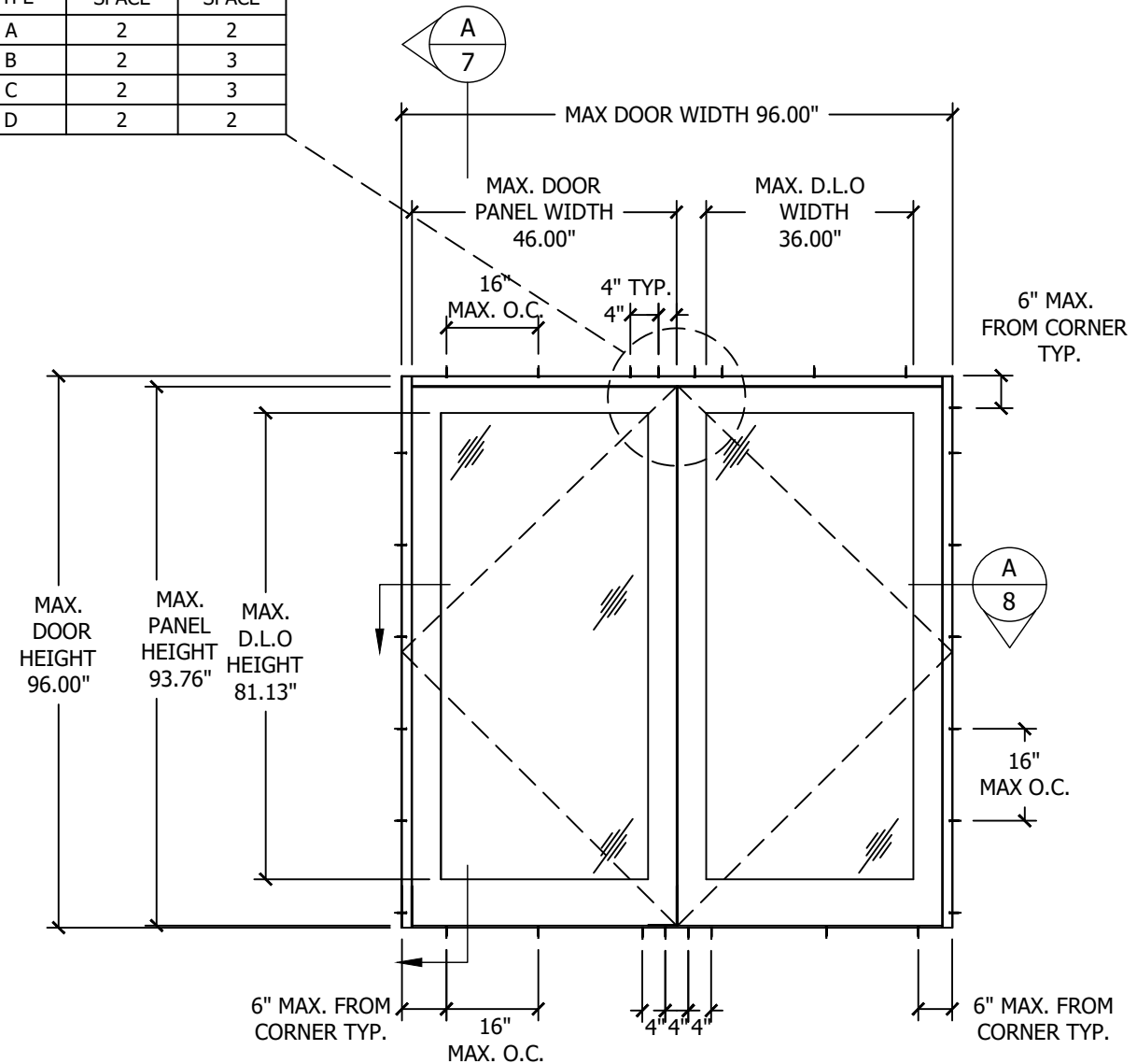
ELEVATION
