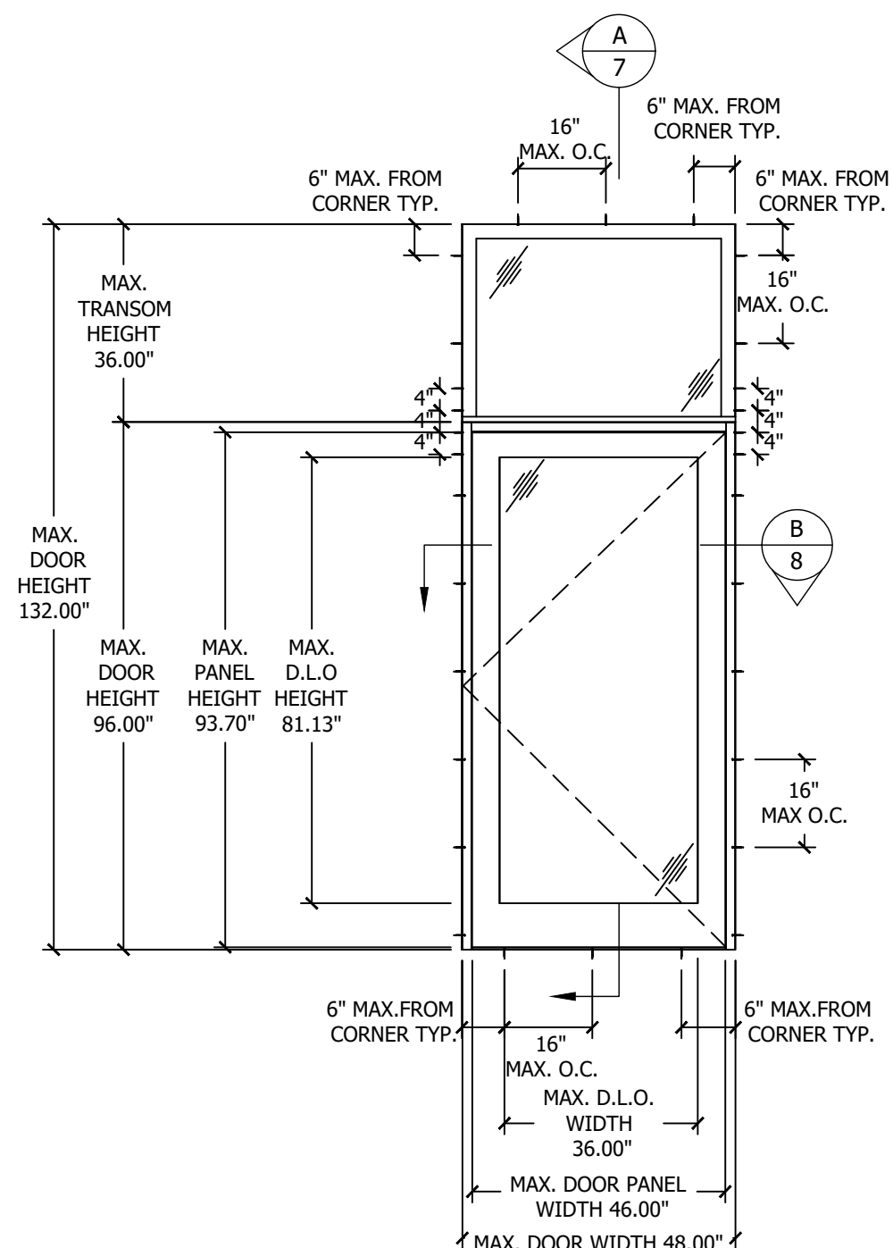
ELEVATION
