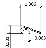
7 600-07 - RAMP
