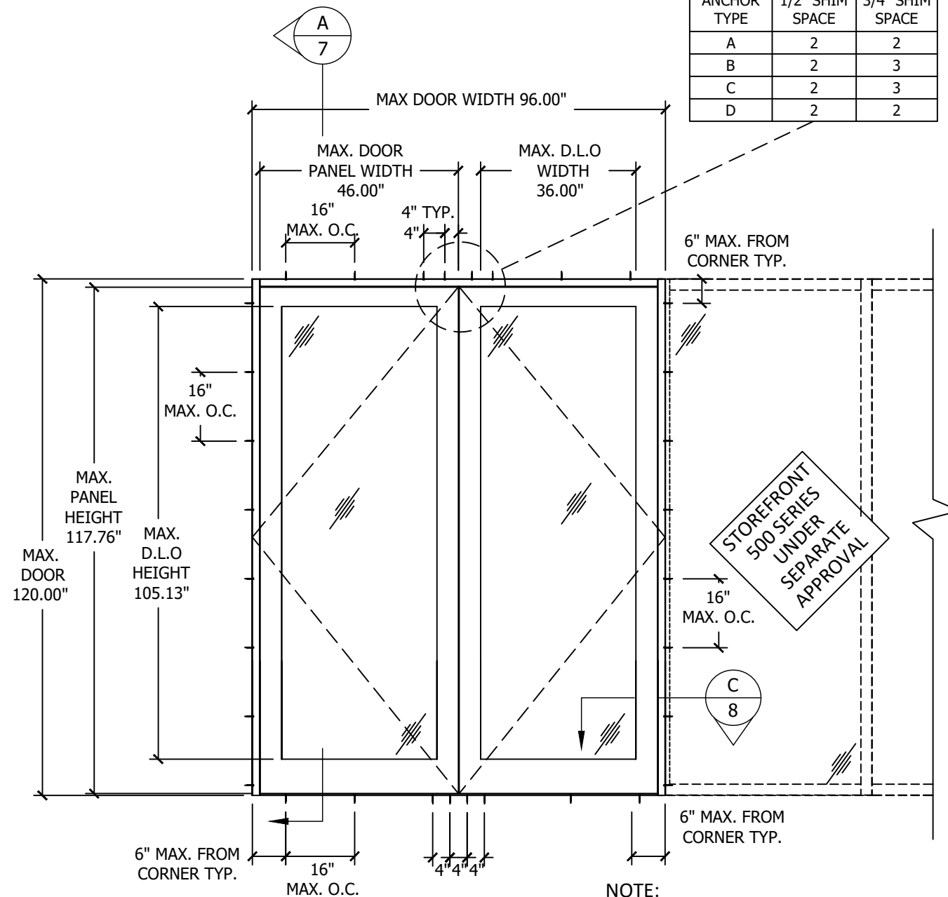
ELEVATION
