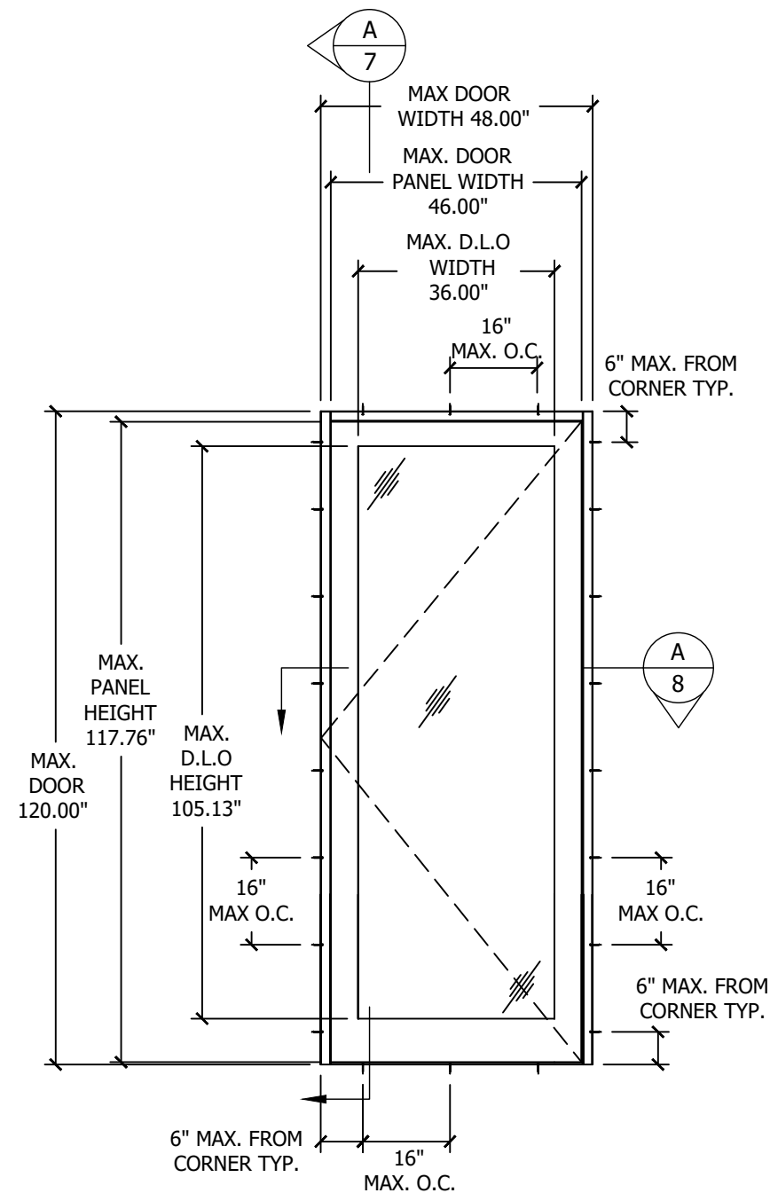
ELEVATION
