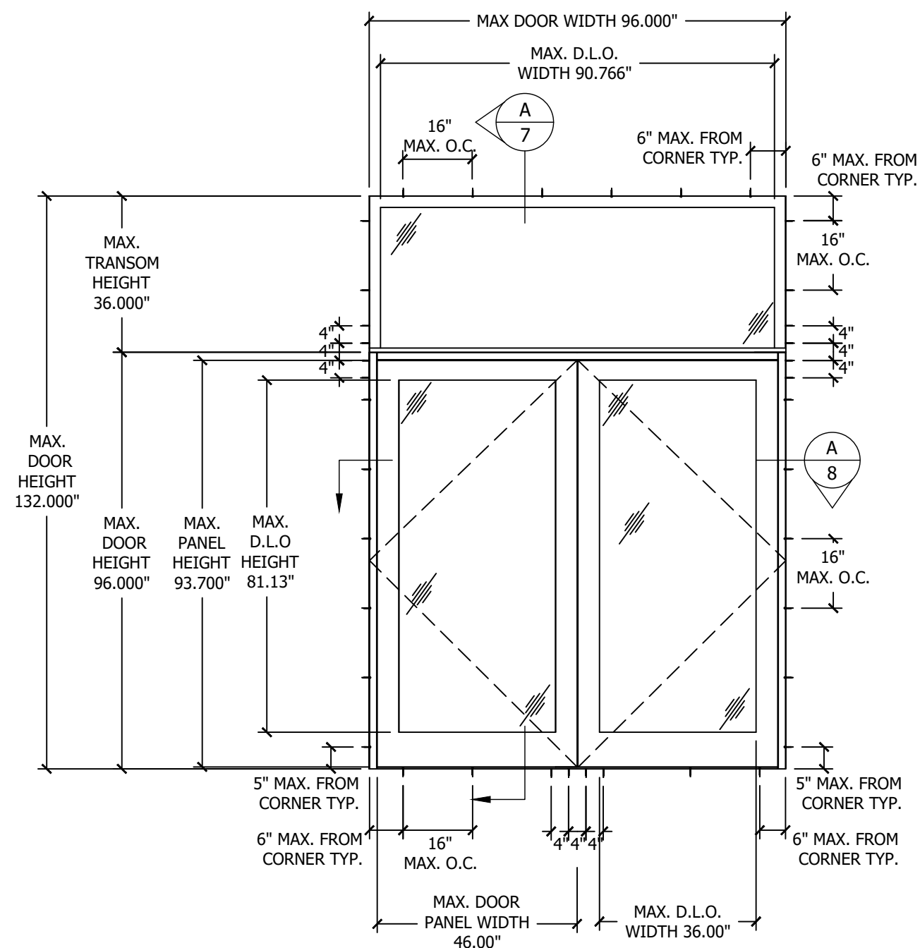
ELEVATION
