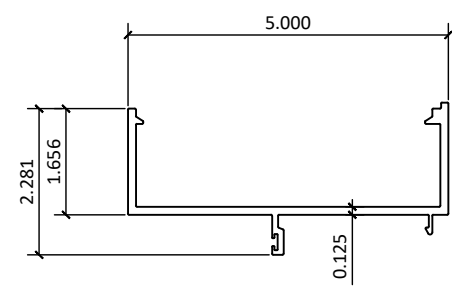
1 600-01 - JAMB
