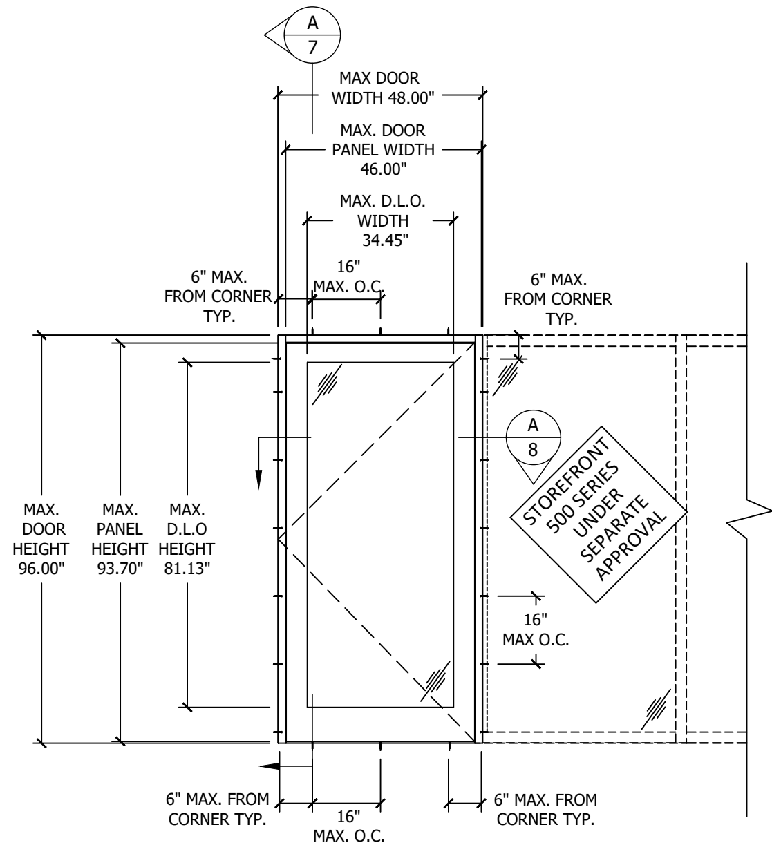
ELEVATION
